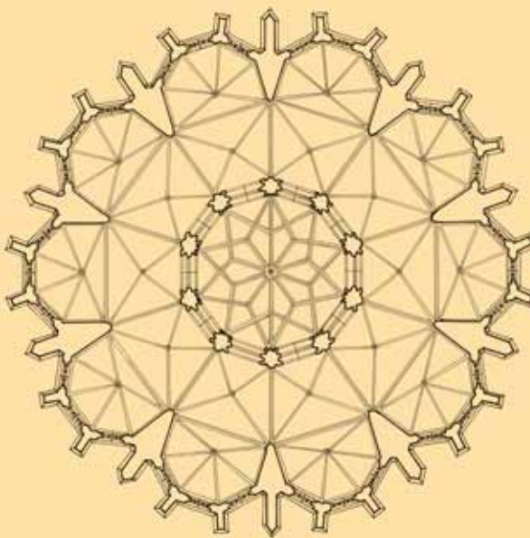
Transformace půdorysu závěru pražské katedrály do podoby dokonalé centrály
