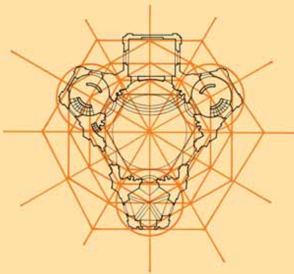
Panenské Břežany, kaple sv. Anny, půdorys, analytický výkres
