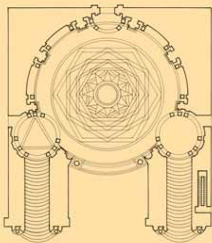
Turin, kaple Sta Sindone, půdorys
