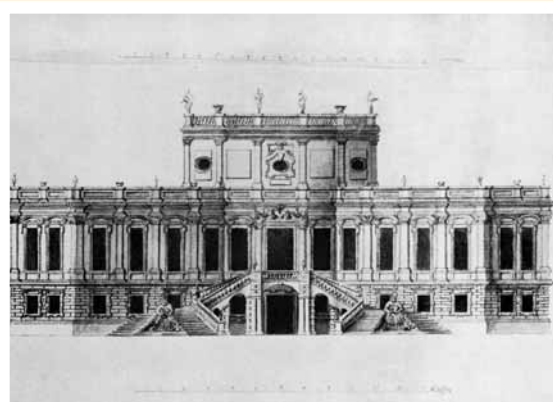
Johann Bernard Fischer von Erlach, letohrádek hraběte Althana v Rossau, výkres průčelí
