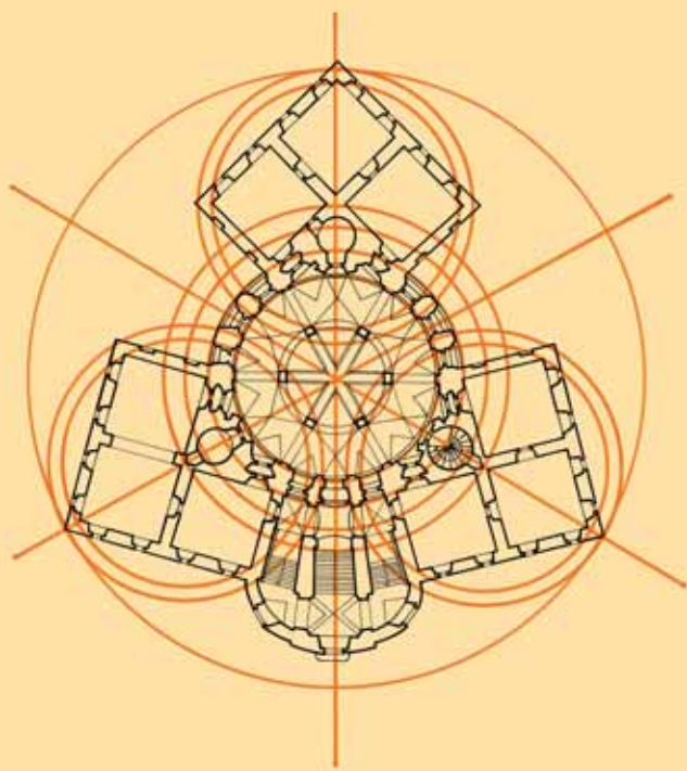
Chlumec nad Cidlinou, zámek Karlova Koruna, půdorys, analytický výkres
