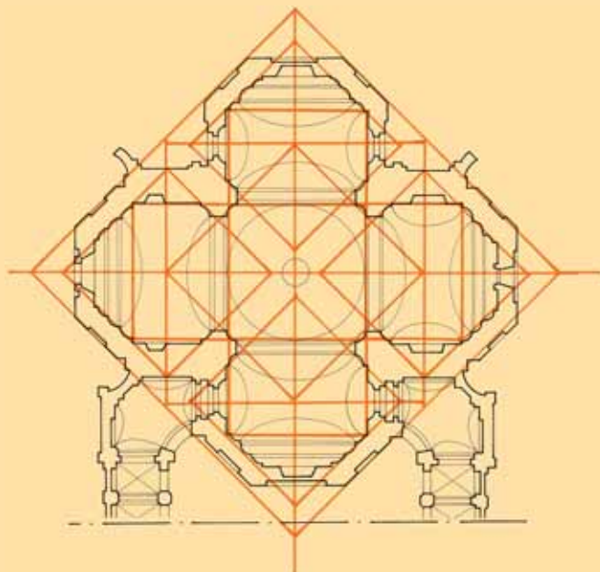
Mariánská Týnice, půdorys kostela, analytický výkres
