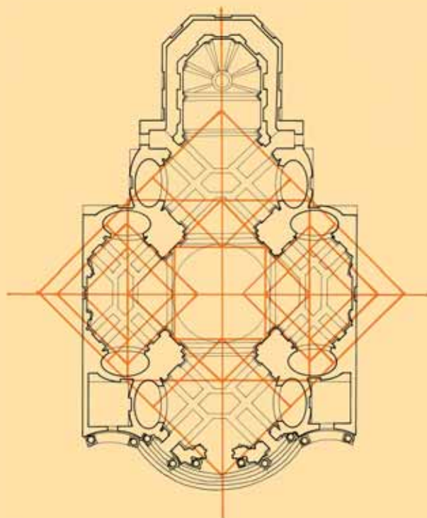
Paříž, návrh Guarina Guariniho pro theatinský kostel sv. Anny, půdorys, analytický výkres
